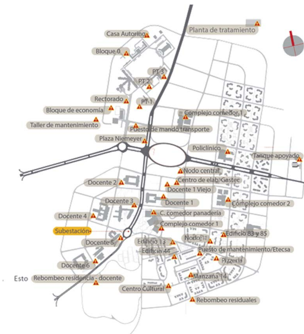
Fig. 7. Plano de grupos electrógenos. Fuente: Rodríguez, 2013.
