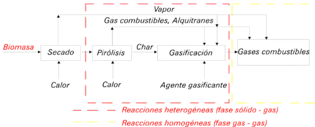
Fig. 1. Secuencia del proceso de gasificación.
