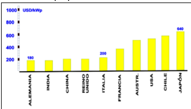
Fig. 6. Restsoftcost por países.
