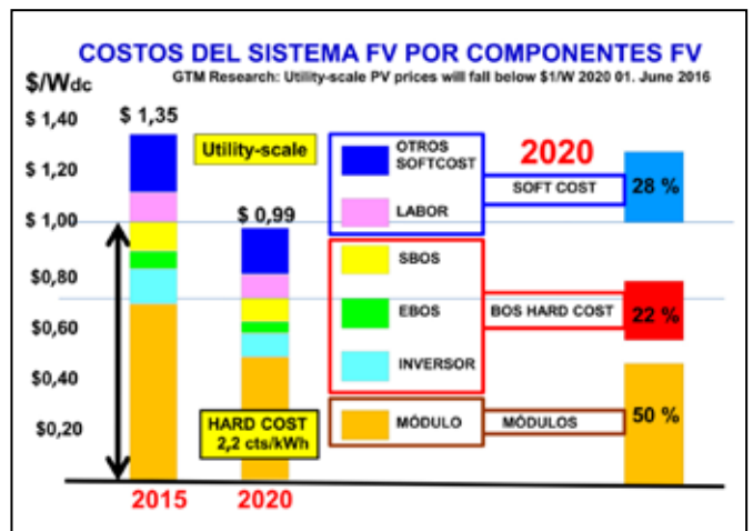
Fig. 10. Costos y pronósticos FV hasta 2020 de la GTM.
