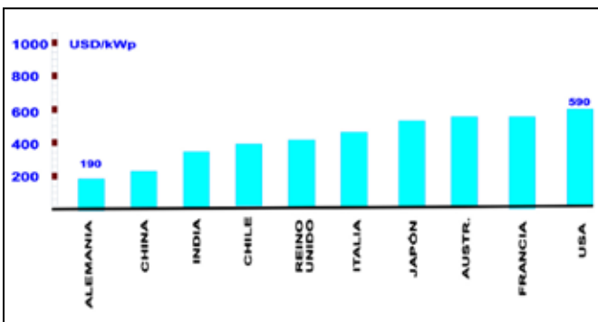
Fig. 4. Otros hardcost «utility» por países. Fuente: Irena Renewable Cost Database.
