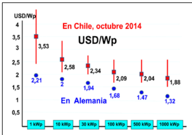
Fig. 11. Costos de Sistemas FV por Wp instalado en Chile y Alemania.
