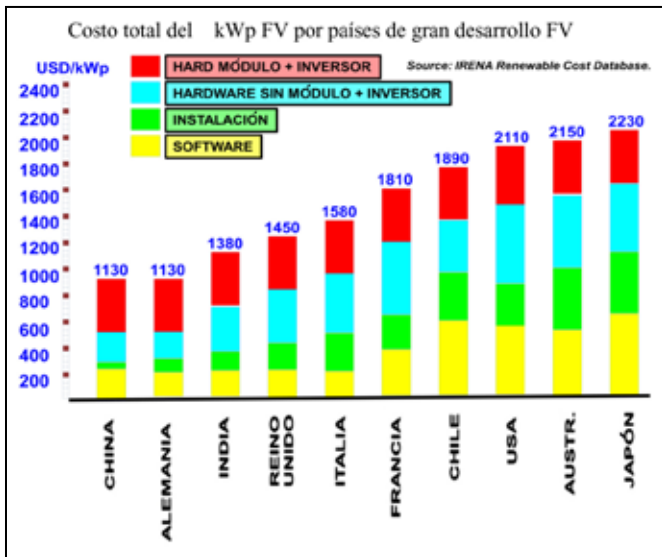
Fig. 8. Costo total del kWp FV por países de mayor desarrollo FV.
