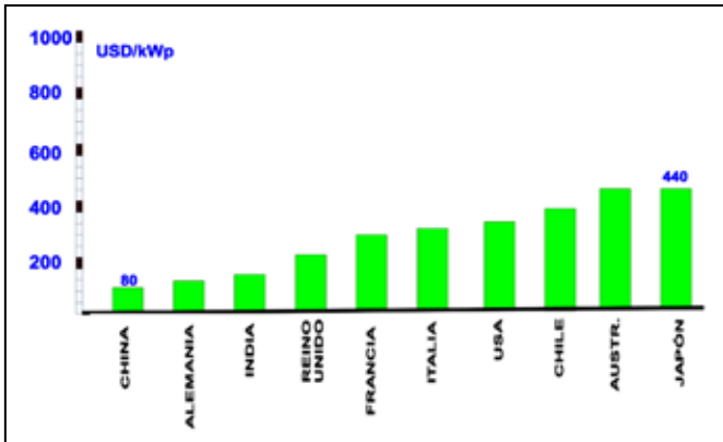
Fig. 5. Softcost instalación por países.
