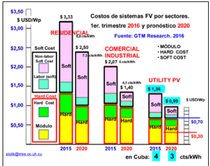
Fig. 16. Aportes de las componentes del sistema a la disminución de los costos totales.
