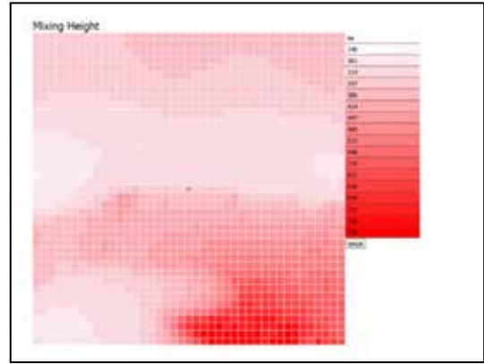
Fig. 7. Representación de la altura de la capa de mezcla.
