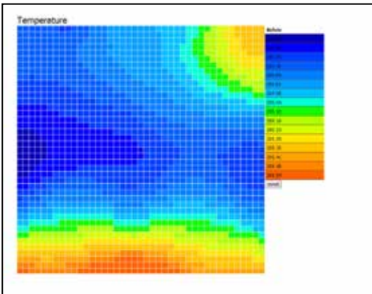
Fig. 5. Representación de la temperatura.
