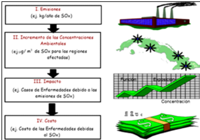
Fig. 2. Metodología Vías de Impacto.
