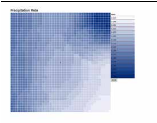
Fig. 6. Representación de la tasa de precipitación.
