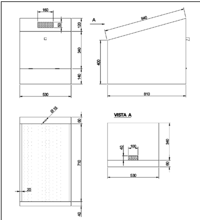
Fig. 3. Planos del secador solar.
