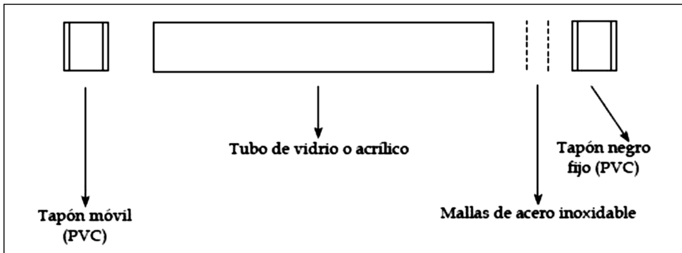
Fig. 1. Esquema de un captador pasivo de NO 2 .
