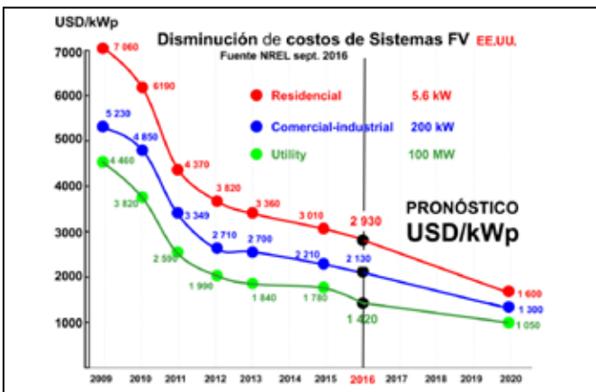
Figs. 14 y 15. Disminución para utility fijo entre 2009 y 2016.
