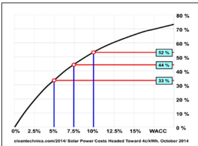
Fig. 9. Aporte del WACC al costo del sistema FV.
