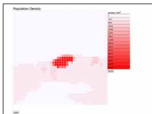
Fig. 13. Representación de la distribución de población en el dominio de la CTE Otto Parellada.
