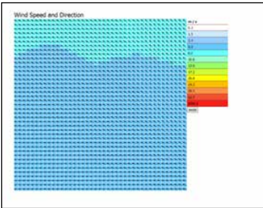
Fig. 4. Representación de la velocidad y dirección del viento.
