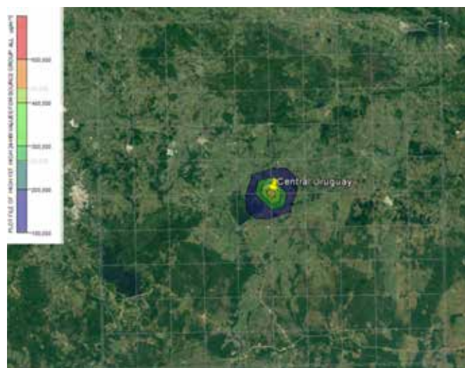
Fig. 5. Isolíneas de concentraciones máximas de PM 10 [ \mu\text{g}/\text{m}^3 ] central Uruguay para 24 horas.
