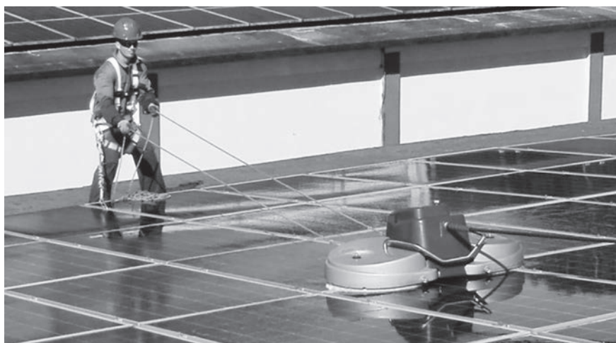
Fig. 1. Instalación de paneles de forma paralela a la cubierta con equipo de limpieza.
