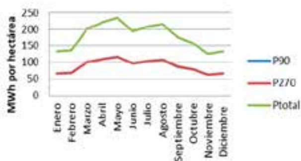
Fig. 5. Producción de un campo a dos aguas con \gamma_1=90 y \gamma_2=270
