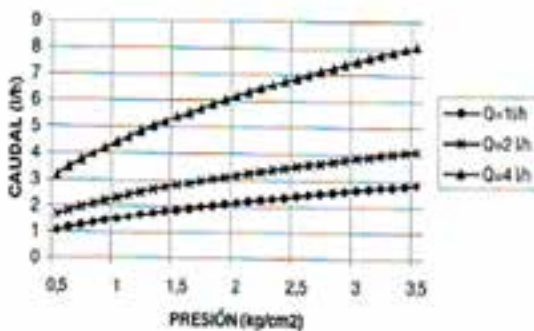
Fig. 1. Caudal de gotero largo D = 16 mm a diferentes presiones.
