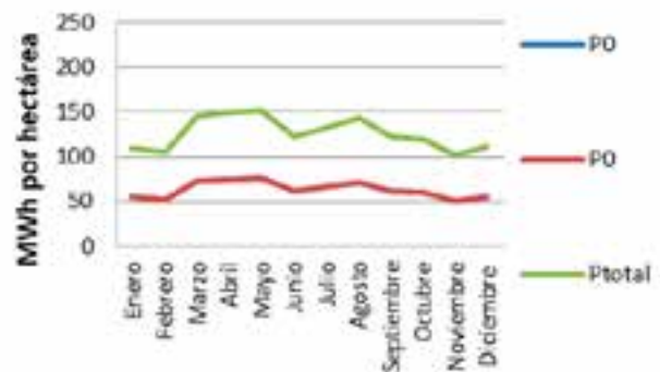
Fig. 1. Producción de un campo orientado al sur con \beta=15^\circ
