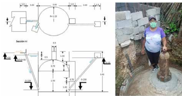
Fig. 1. Diseño e imagen del biodigestor casero en fase de construcción, a manos de su usuaria Marelis Galindo González en tiempos de la contingencia sanitaria. Ella es la primera mujer albañil en el contexto del MUB.
