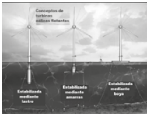
Fig. 3. Eólica marina flotante.
