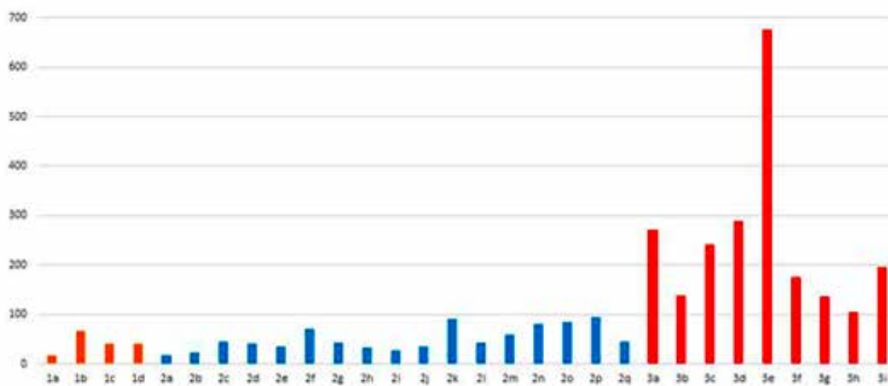
Fig. 12. Consumo de energía final según indicadores de kWh /m²/año en los casos analizados: nZEB clima cálido húmedo (naranja), hoteles europeos nZEB (azules) y hoteles cubanos (rojos). Se utilizó un factor de ponderación de 2,5 para convertir los datos de energía primaria final, en aquellos casos que no se contaba con este valor.
