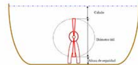
Fig. 2. Esquema frontal del posicionamiento de la turbina.
