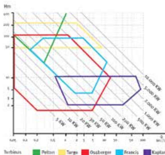
Fig. 1. Curva de rendimiento de cada turbina.
