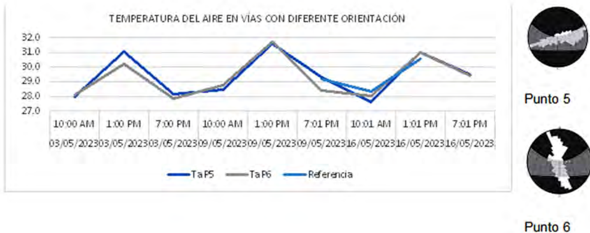
Fig. 7. Temperatura del aire medida en los puntos 5 y 6 ubicados en vías con diferente orientación, y en la referencia externa. Habana Vieja.
