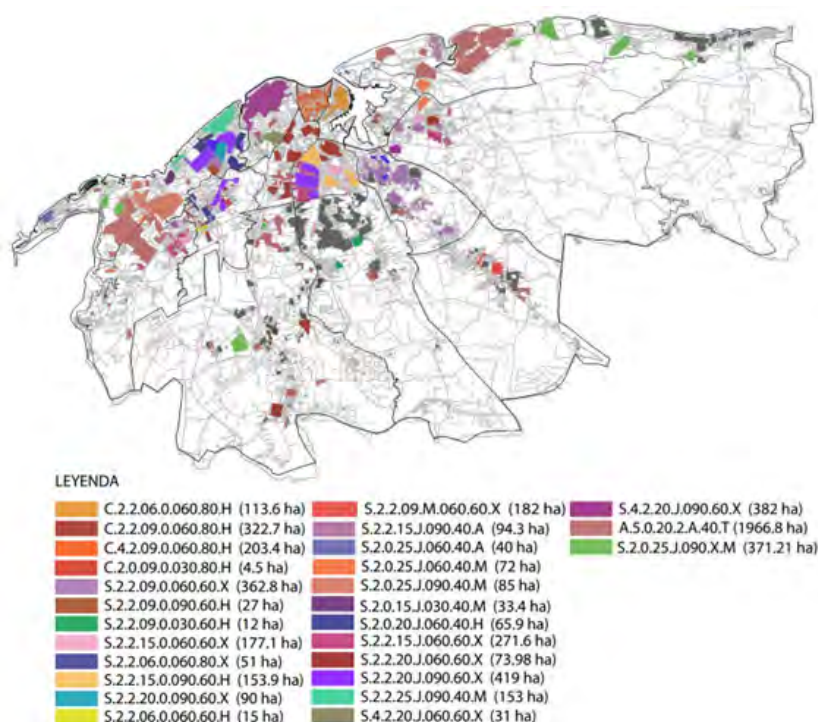
Fig. 1. Tipos morfológicos identificados en La Habana. Fuente: Elaboración propia.
