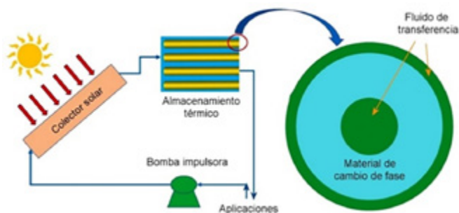
Fig. 1. Sistema de calefacción solar de eficiencia, mejorada con PCM. En este caso la T_f del material es cercana a la temperatura ambiente.
