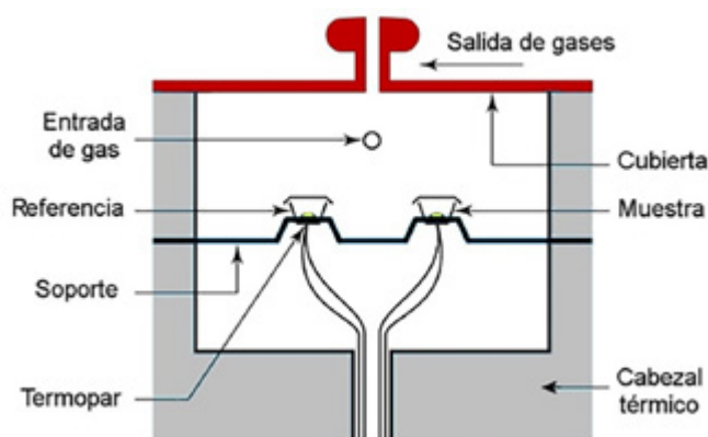
Fig. 4. DSC mediante flujo de calor (HF DSC).
