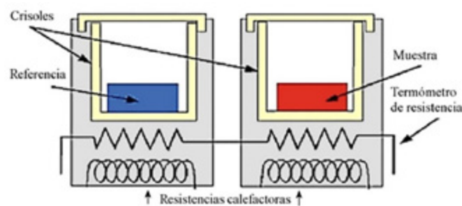
Fig. 6. DSC por compensación de potencia (PC DSC).
