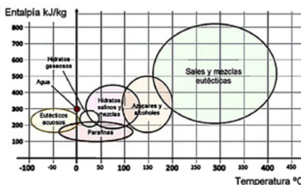
Fig. 3. Intervalos de temperatura de trabajo de diversas sustancias PCM.
