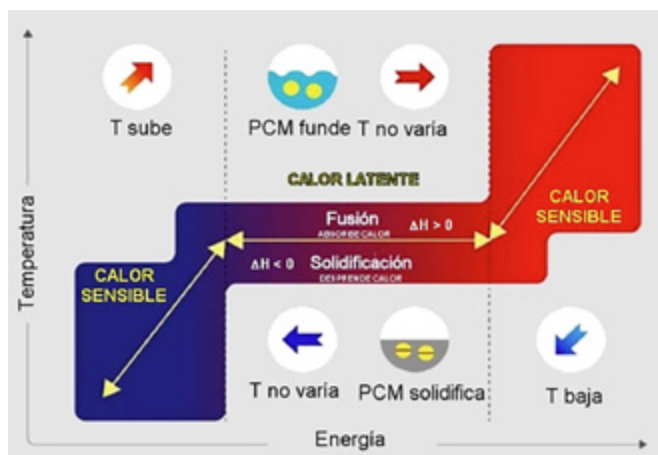
Fig. 2. Comportamiento de un material PCM al variar la temperatura. La temperatura de fusión se escoge de acuerdo con la temperatura que se desea regular.
