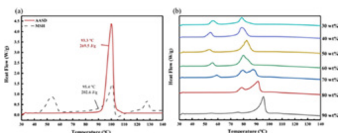
Fig. 7. A la izquierda, curvas DSC de los sulfatos puros: AASD, sulfato doble de aluminio y amonio; MSH, sulfato de magnesio. A la derecha, mezcla de ambos a partir del sulfato doble.
