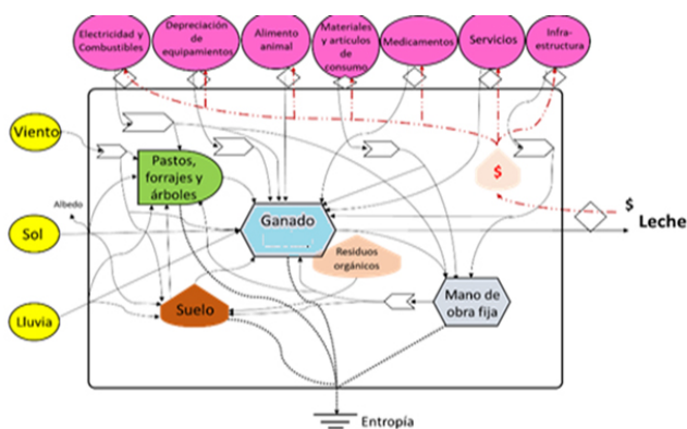
Fig. 1. Diagrama simplificado del flujo de energía en la unidad caprina.
